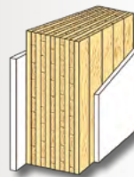
Außenwand 11 Lagen entspricht 25,0 cm
