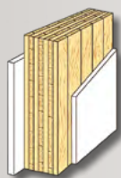
Innenwand 7 Lagen entspricht 16,0 cm
