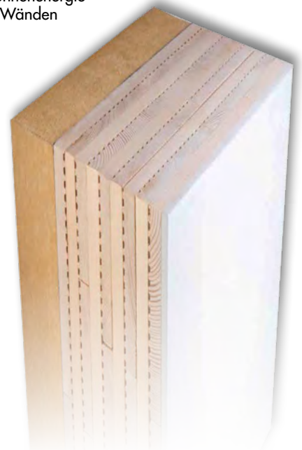
Außenwand 11 Lagen entspricht 25,0 cm
