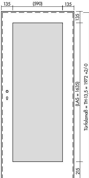
LA mit flächenbündigem Leistenrahmen
