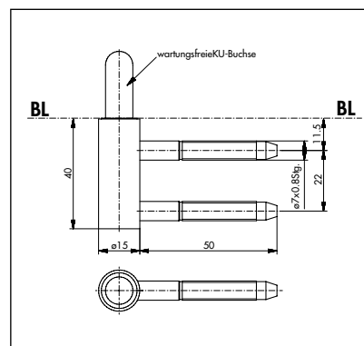
Rahmenteil für Holzzargen wartungsfrei
