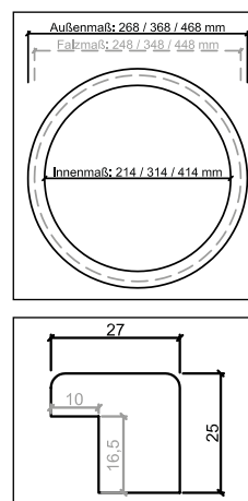
Maße vom Bullaue
