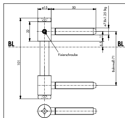
Flügelteil wartungsfrei, 3-teiliges Band mit Sicherungsstift
