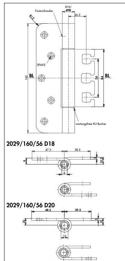
2029/160/56 D18 und 2029/160/56 D20 für stumpfe Türen
