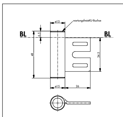
Rahmenteil für Stahlzargen wartungsfrei, 3-teiliges Band, 26 mm
