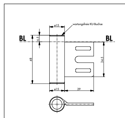
Rahmenteil für Stahlzargen wartungsfrei, 3-teiliges Band, verlängerter Lappen, 29 mm
