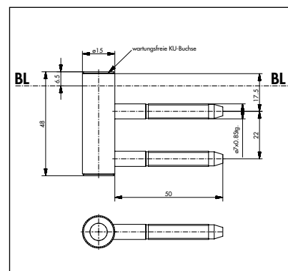
Rahmenteil für Holzzargen wartungsfrei, 50 mm
