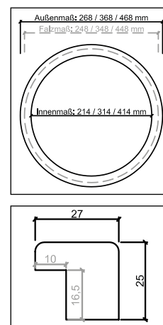
Maße vom Bullaue
