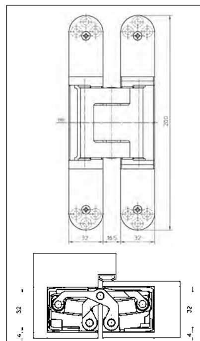
TECTUS TE 540 3D für stumpfe Türen bis 120 kg
