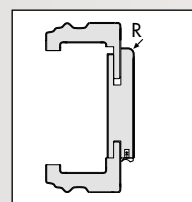
PZ-4 R Ausführung profilierter Beklei- dungen, runde Futterplatte
