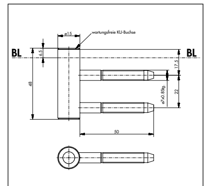
Rahmenteil für Holzzargen wartungsfrei, 50 mm
