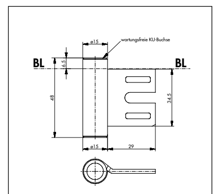
Rahmenteil für Stahlzargen wartungsfrei, 3-teiliges Band, verlängerter Lappen, 29 mm
