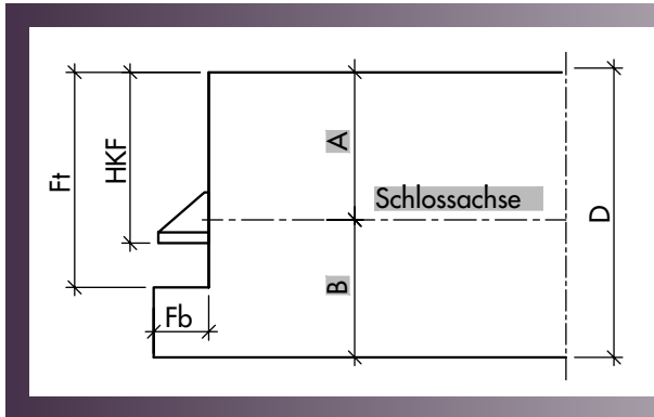
Türblatt gefälzt (alle Maße in mm)
