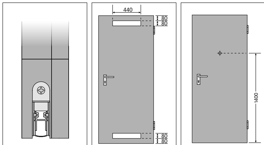
Bodendichtung
