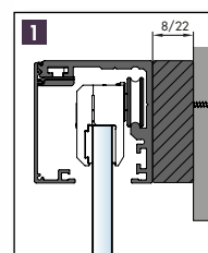
Adapterleiste
