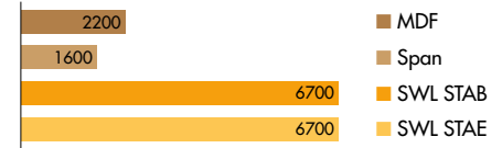
Elastizitätsmodul quer (N/mm 2 )
